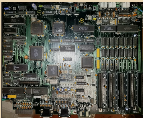
Рис. 7. Материнская плата Tandy 1000 с микросхемой Tandy Sound NCR 8496PT ( U7 в верхнем ряду микросхем). Правее – разъём J1 для подключения системного динамика (на него кроме системных звуков выводились звуки Tandy Sound), наушников J2 , регулятор громкости
