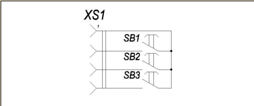
Рис. 4. Схема выносного пульта регулировки громкости
