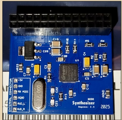
Dream SAM2695 крупным планом. Современная микросхема синтезатора изготовлена в корпусе QFN48 размером всего 6x6 мм (шаг между ножками – 0.4 мм!), поэтому данная «дочка» самая маленькая
