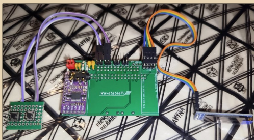
Рис. 10. Wavetable-Pi с подключёнными кнопками и дисплеем
